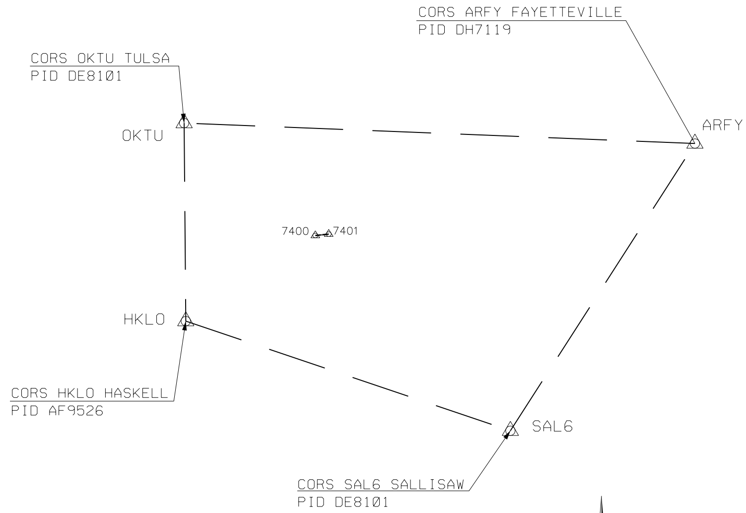
UTILIZED CORS STATIONS N.T.S.
