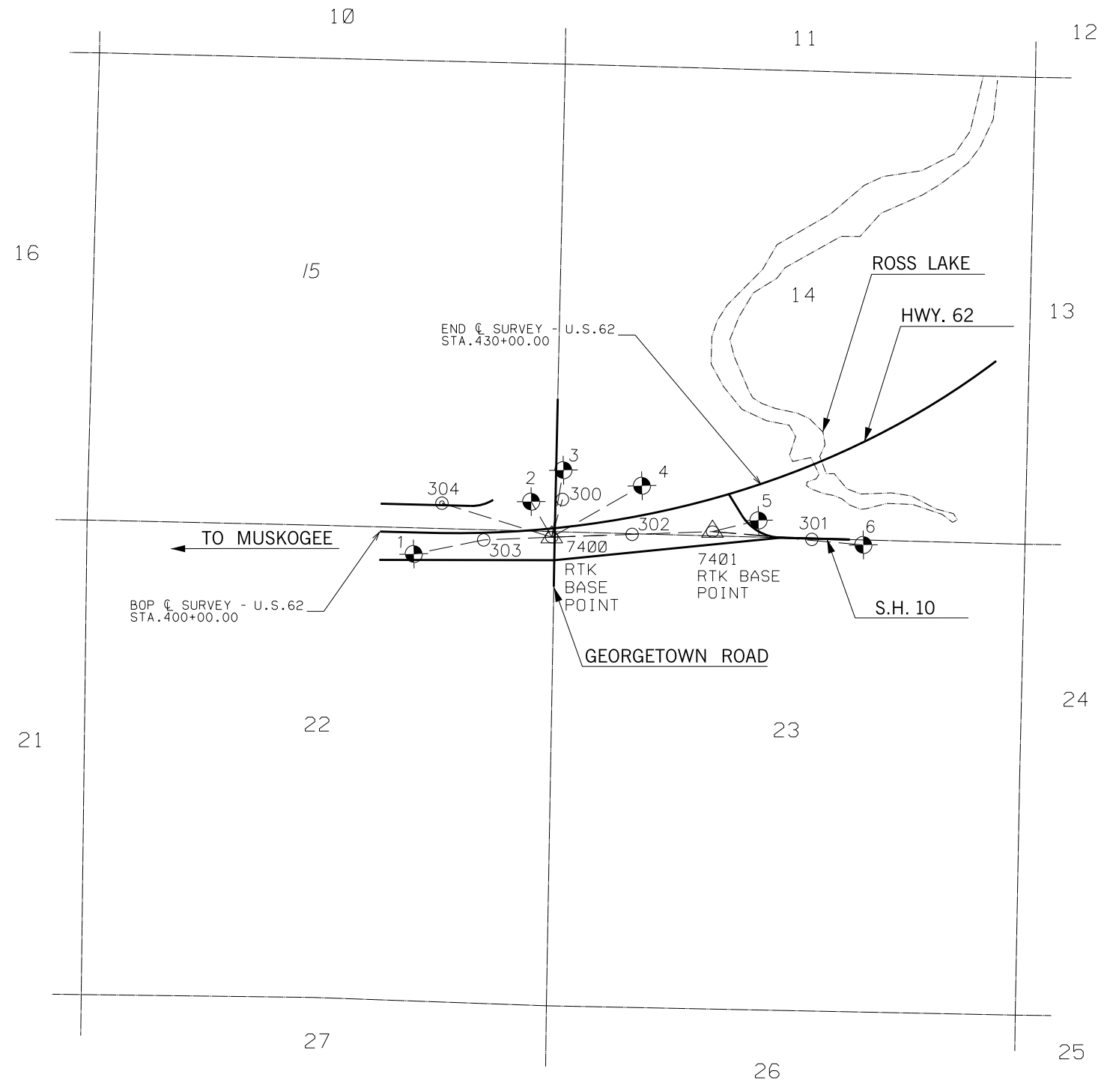
HORIZONTAL CONTROL DIAGRAM N.T.S.
